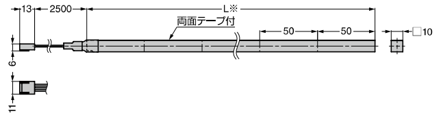
※長さは50 mmピッチで調節できます。
