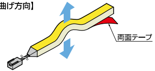
両面テープ貼付面に対して、垂直方向に曲がります。水平方向には曲がりません。
