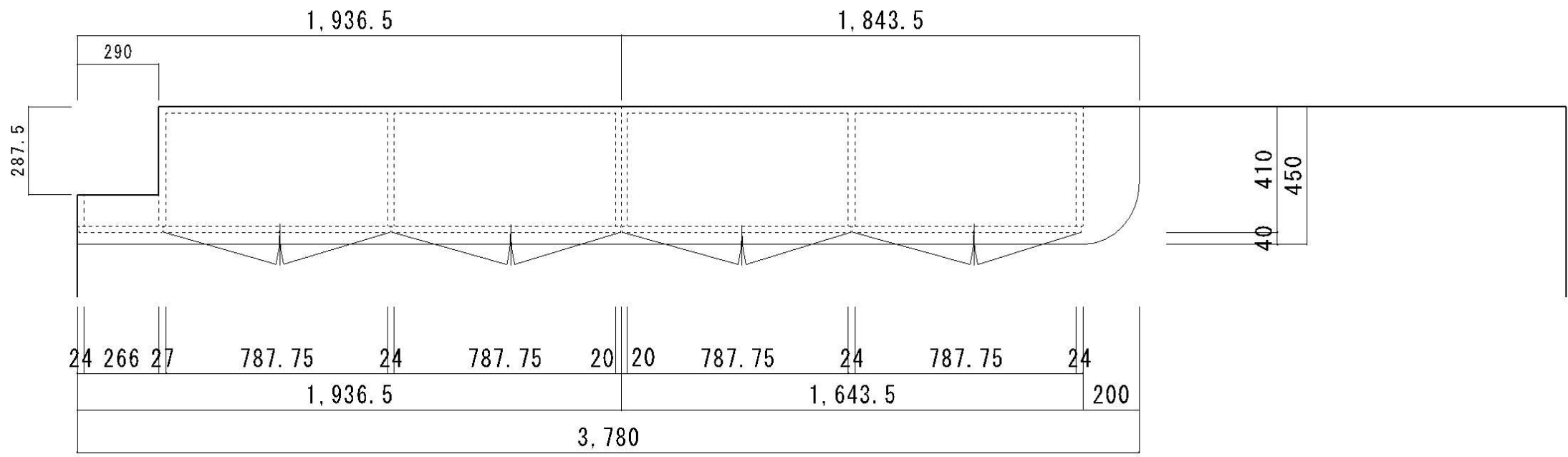
平面図 S=1/20
